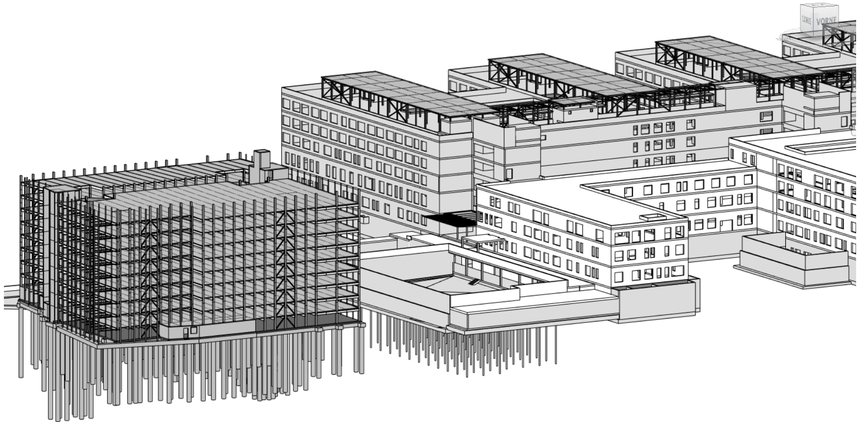
Screenshot | Statikmodell | Gründung | Parkhaus West, Wirtschaftshof
